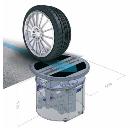
Bild 2: Über Laserdioden-Digitalkameras, die in Fahrbahn-Schächten oder U-Rinnen eingelassen sind, werden Reifenprofile in Millisekunden aufgezeichnet und vom integrierten Hutschienen-PC Kontron ThinkIO berechnet.
